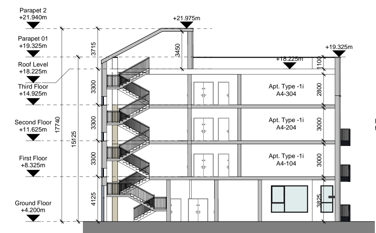
B Section BB 1 : 200
