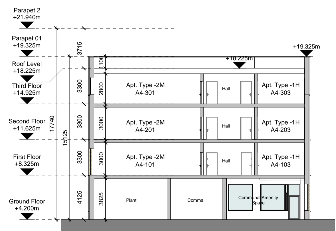
A Section AA 1 : 200
